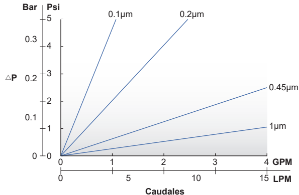
10" Cartucho Filtro Plisado de Membrana de PVDF
