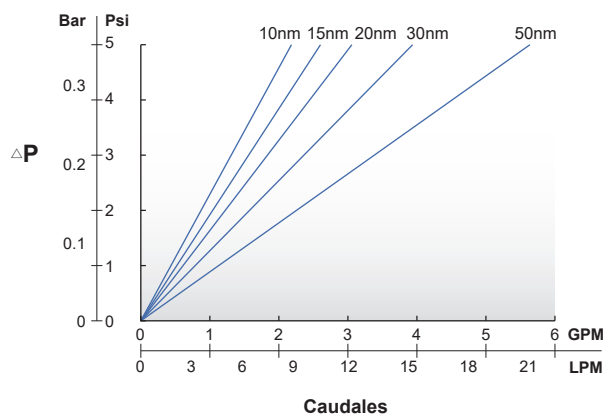
10" Cartucho Filtro Plisado de Membrana de Nilón
